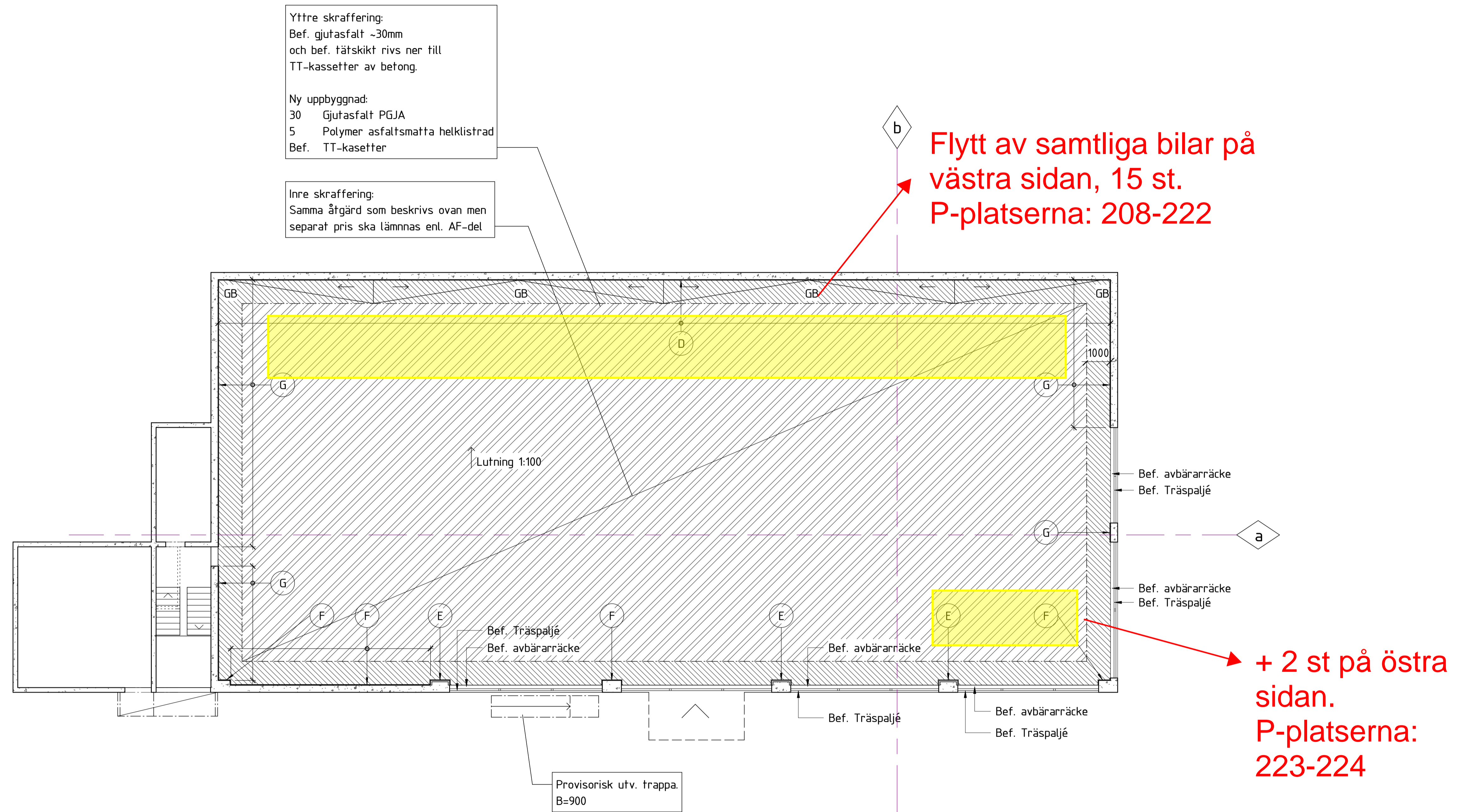
Plan 2 1:100
